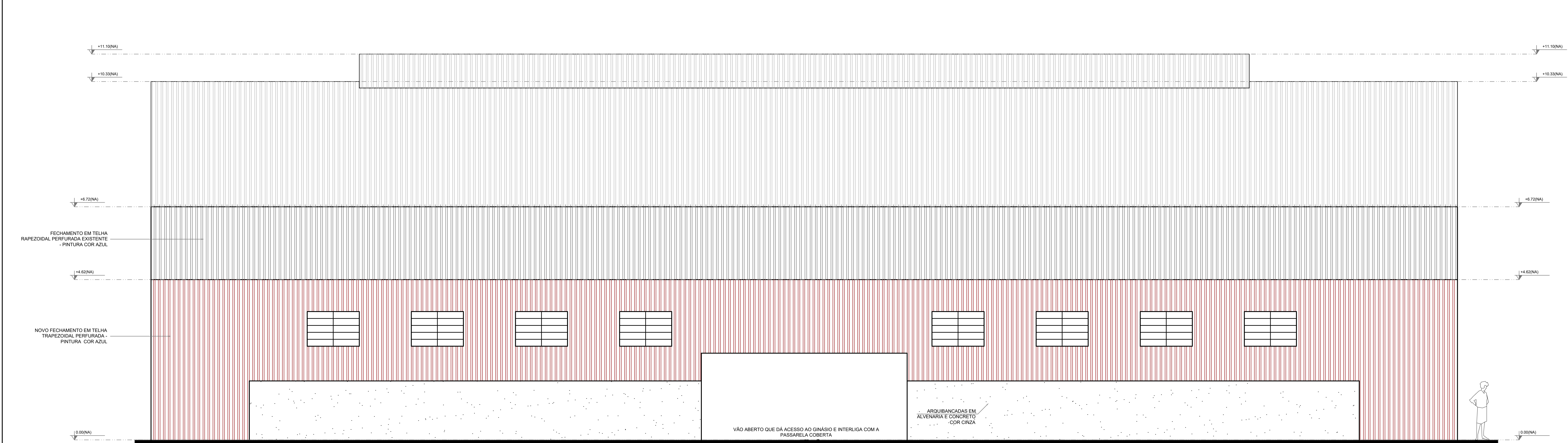
2 Fachada Lateral 04 - Estrutura Metálica ESCALA 1/50
