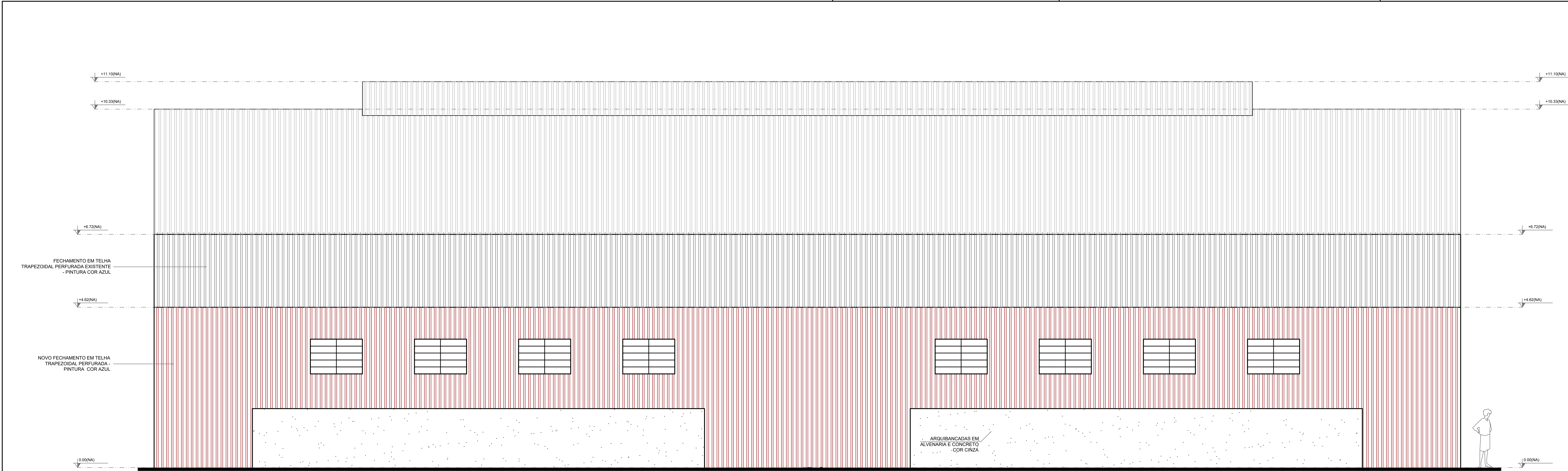
1 Fachada Lateral 03 - Estrutura Metálica ESCALA 1/50
